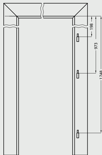
Vodorovný rez
