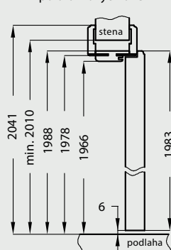
vyžadovaná výška otvoru ve zdi 2010 mm
