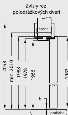
vyžadovaná výška otvoru ve zdi 2010 mm
