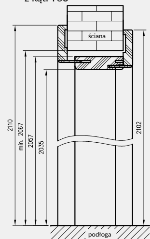
Przekrój pionowy tunelu regulowanego z ką. T63
