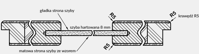
Przekrój poziomy drzwi VETRO B5, B10-B11
