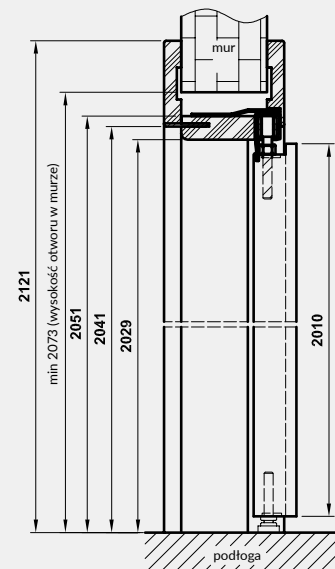
Przekrój pionowy
